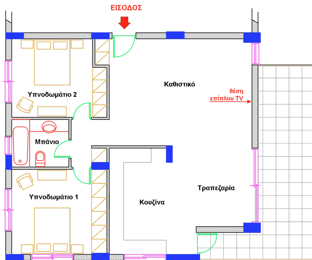
ΚΑΤΟΨΗ ΔΙΑΜΕΡΙΣΜΑΤΟΣ ΚΛΙΜΑΚΑ 1:100
