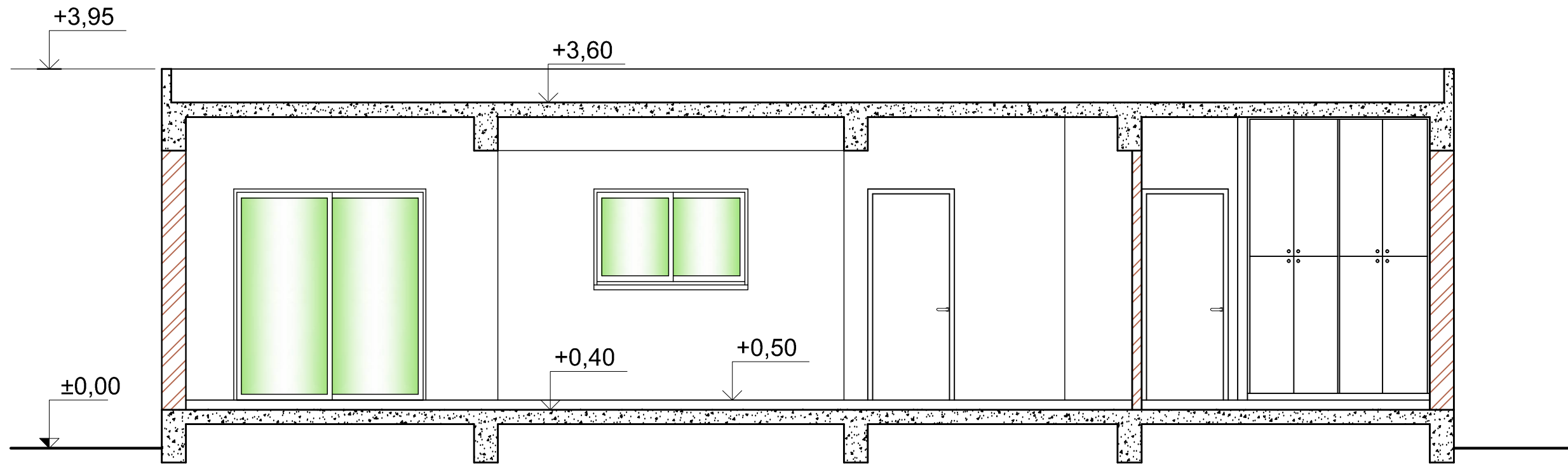
ΤΟΜΗ Α - Α ΚΛ. 1:50
