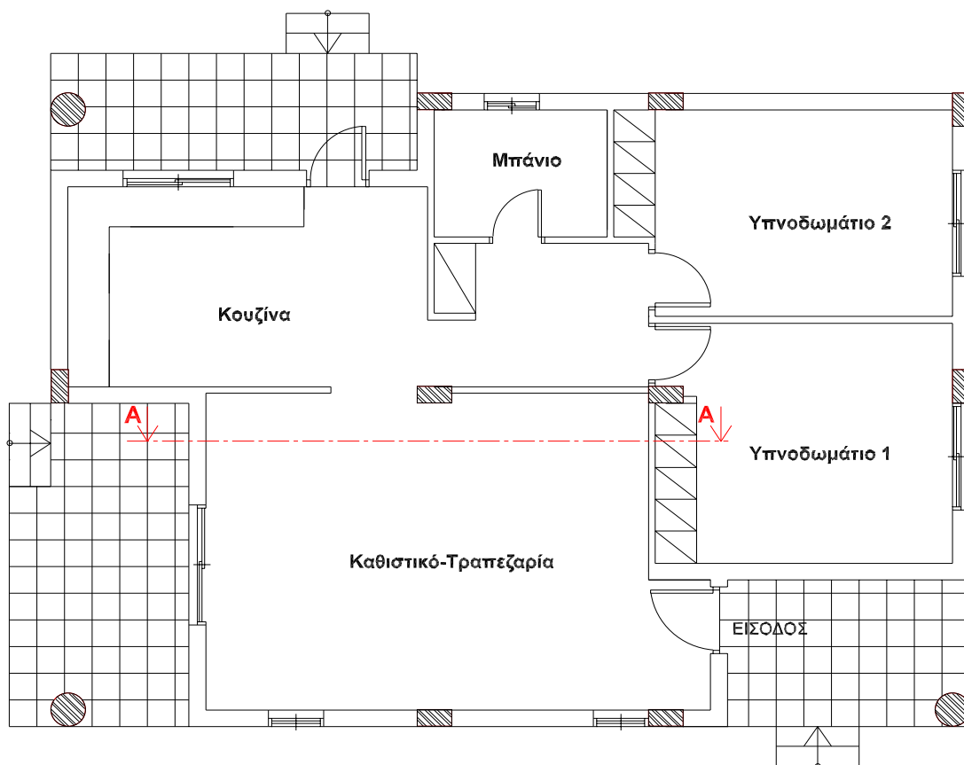
Κάτοψη Κατοικίας ΚΛΙΜΑΚΑ 1:00
