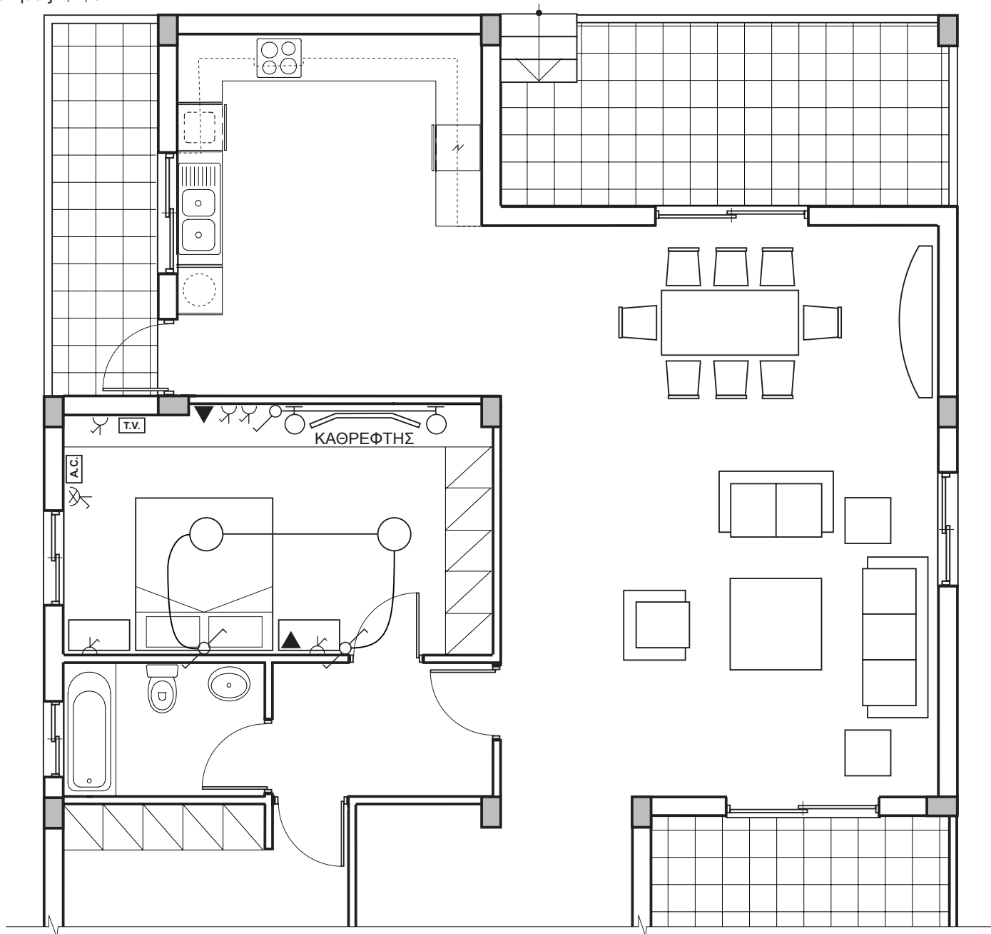
ΚΑΤΟΨΗ ΙΣΟΓΕΙΟΥ ΚΛ. 1:50 ΣΧΗΜΑ 1
