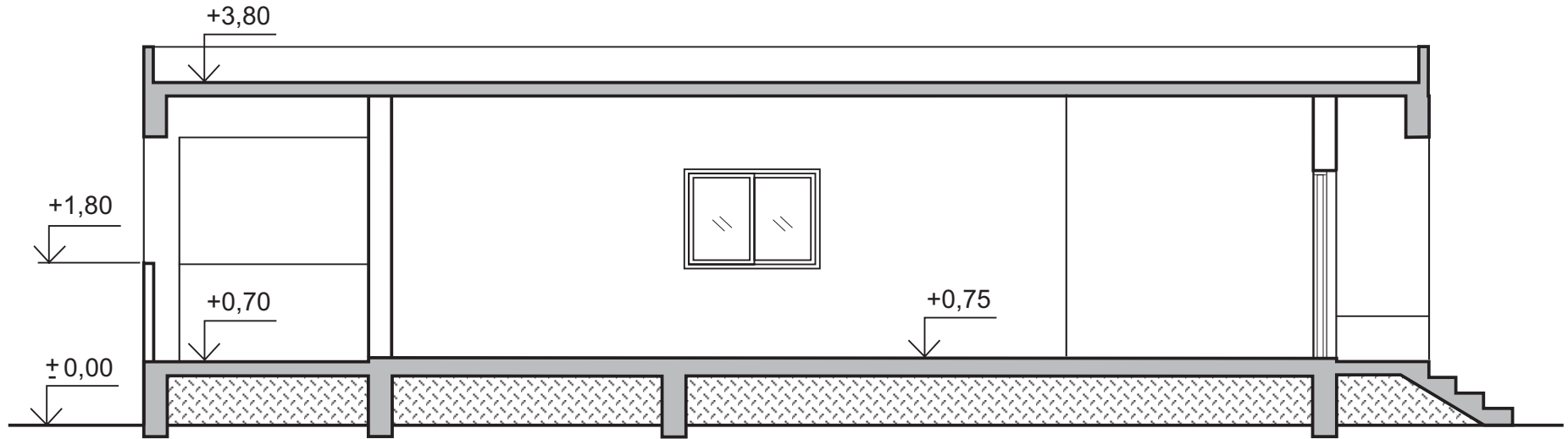
ΤΟΜΗ Β-Β ΚΛ. 1:50
