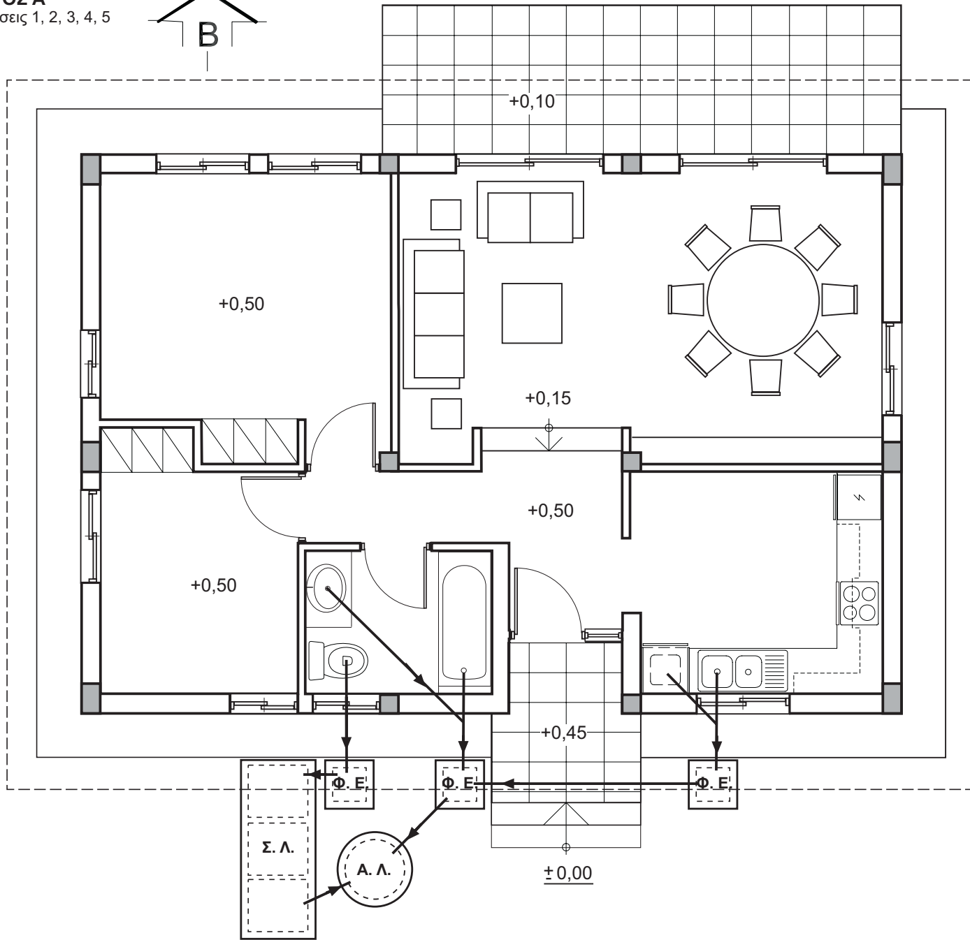
ΚΑΤΟΨΗ ΙΣΟΓΕΙΟΥ ΚΛ. 1:50 ΣΧΗΜΑ 2
