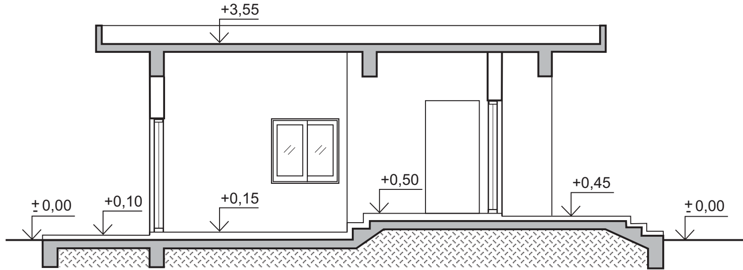
ΤΟΜΗ Β-Β ΚΛ. 1:50
