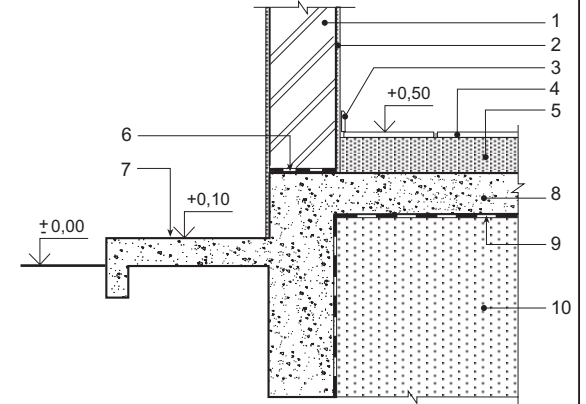
ΚΑΤΑΣΚΕΥΑΣΤΙΚΗ ΛΕΠΤΟΜΕΡΕΙΑ Β ΚΛ. 1:20
