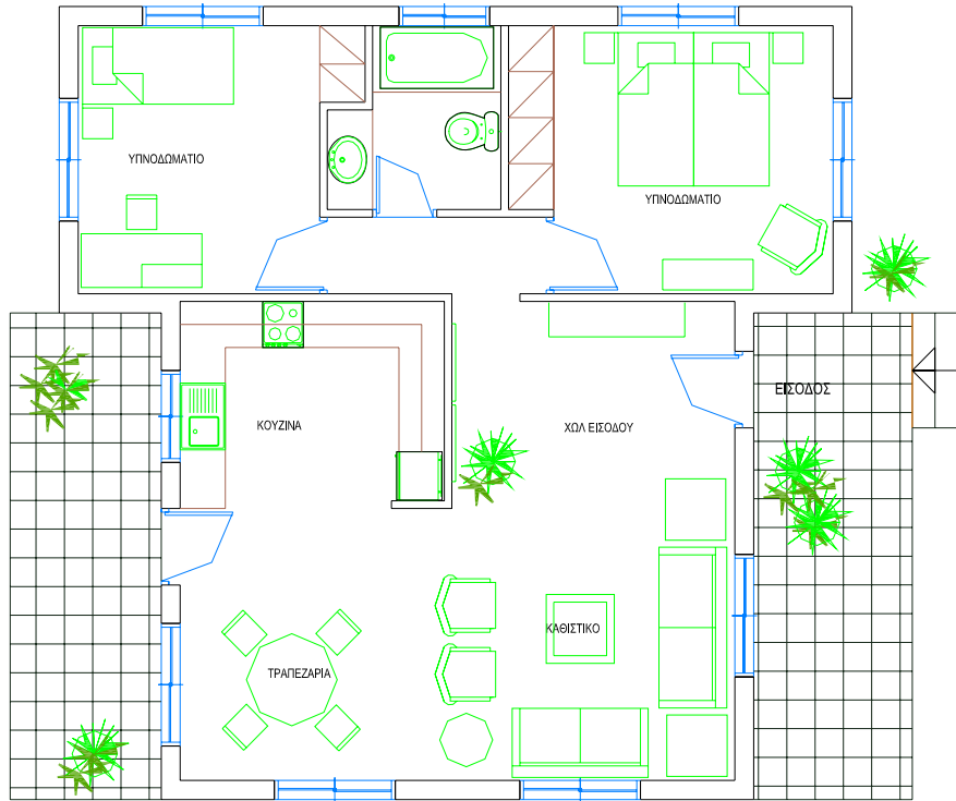
ΚΑΤΟΨΗ ΚΑΤΟΙΚΙΑΣ ΚΛΙΜΑΚΑ 1:50
